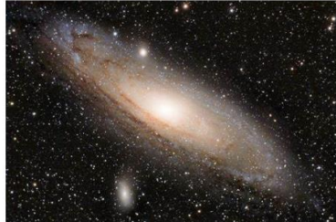
Galaxia de Andr6meda
